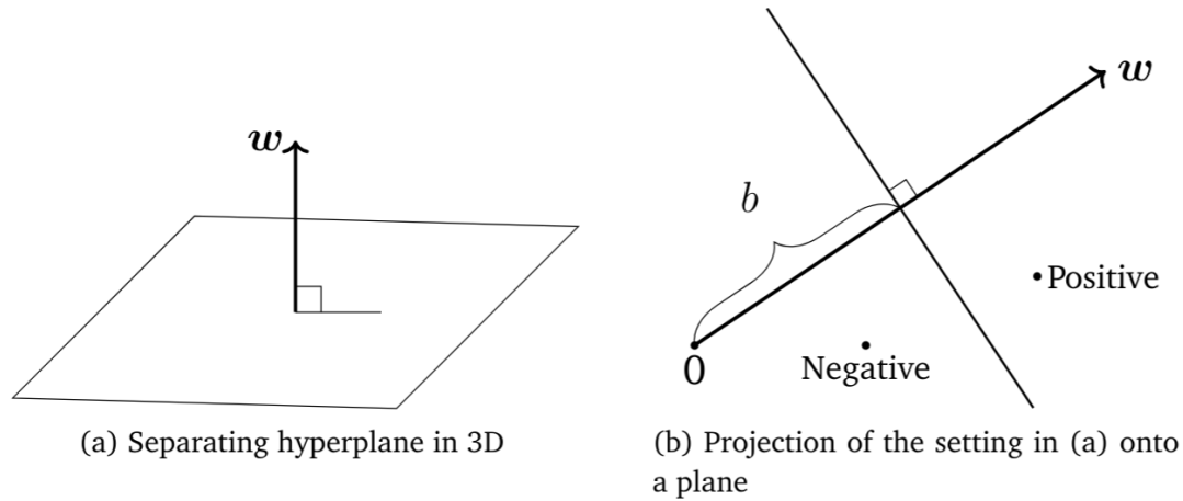
Figura 8.1: (a) Iperpiano separatore in uno spazio tridimensionale, con il vettore normale w perpendicolare all'iperpiano. (b) Proiezione bidimensionale della configurazione: l'intercetta b rappresenta la distanza firmata dall'origine all'iperpiano, mentre il segno di f(x) indica se un punto appartiene alla classe positiva o negativa.
