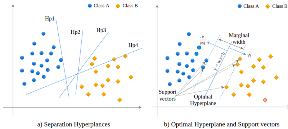
Figura 8.2: (a) Esempio di diversi iperpiani che separano le due classi lineari (Class A e Class B). (b) Iperpiano ottimale trovato dalla SVM, con i vettori di supporto evidenziati e la larghezza del margine determinata dalla distanza tra i due iperpiani paralleli.
